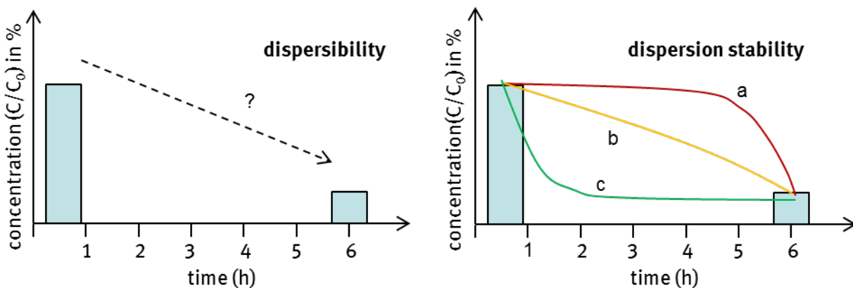
Abbildung 1: Mögliche Ergebnisse aus dem Dispergierbarkeits- und Dispersionstabilitätstest, das 2-Punkt und 7-Punkt Messverfahren.
